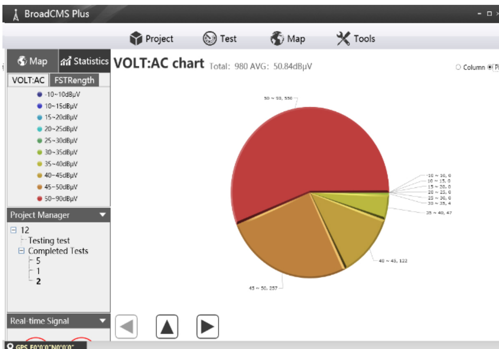
图 5 饼图示意图
